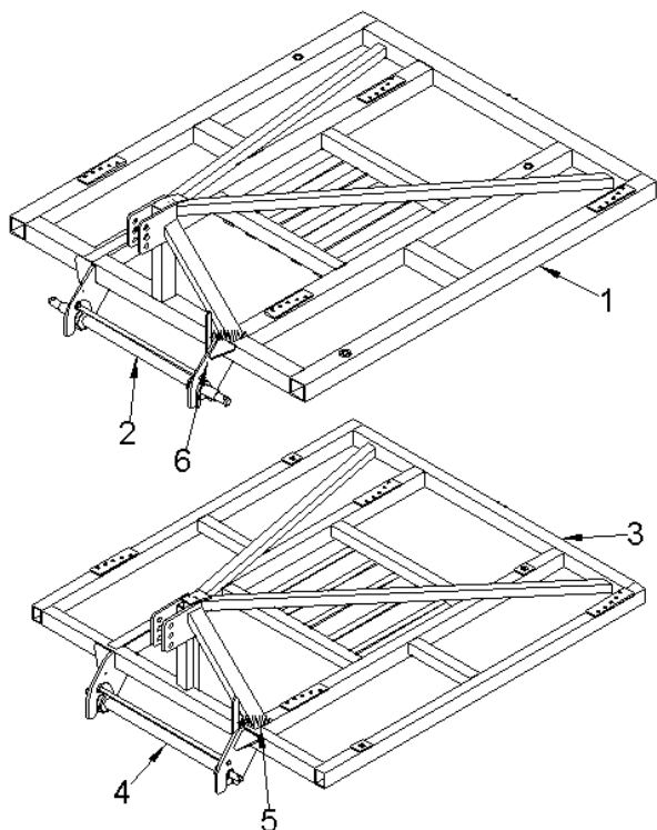
Výkres č.8 Rám stroje (tabulka 8)
