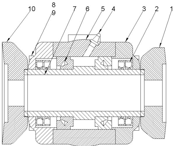
Výkres č.11 Sestava domečku ložiska (tabulka č.11)
